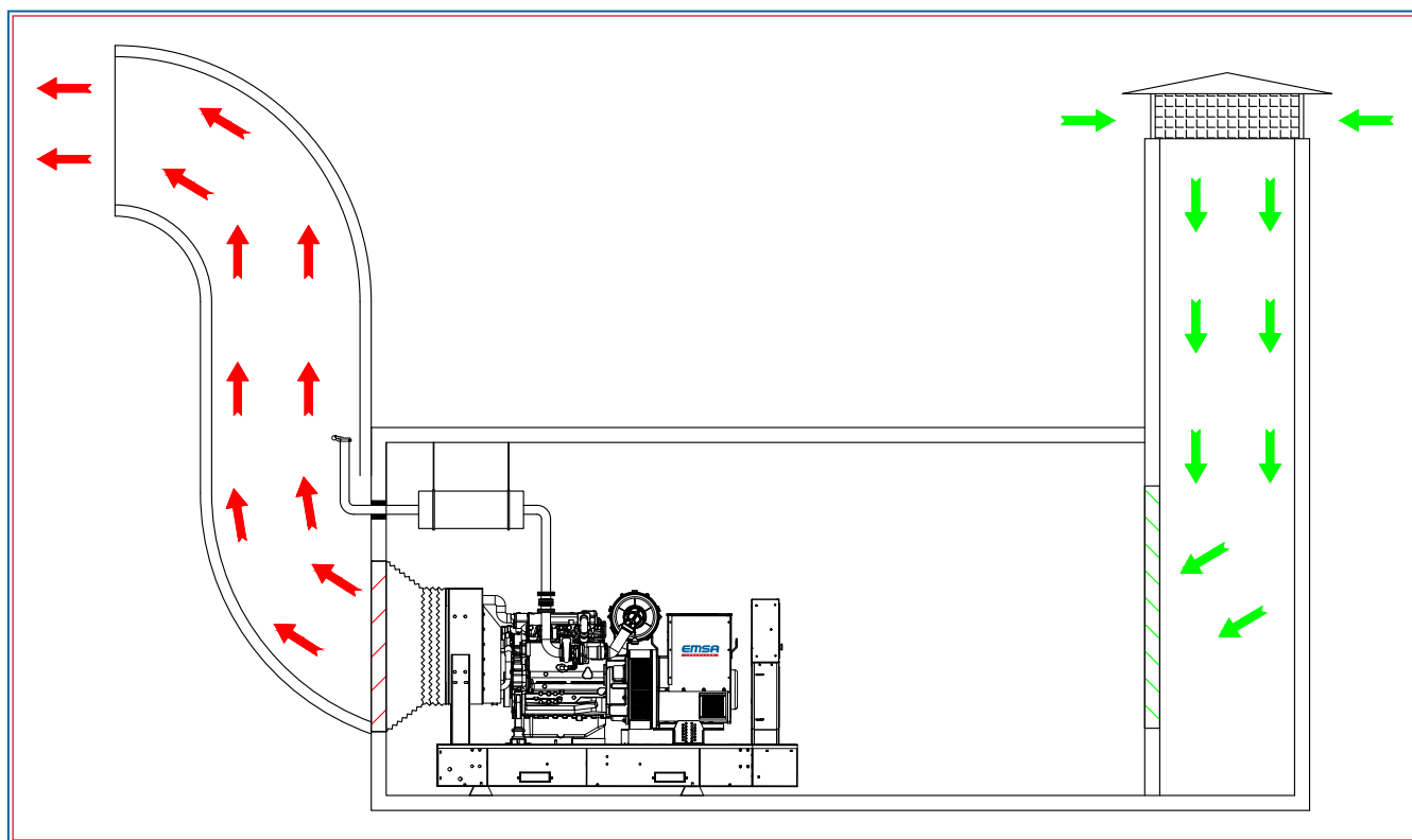
Рисунок-9 Типичный план размещения генератора в подвальном помещении
