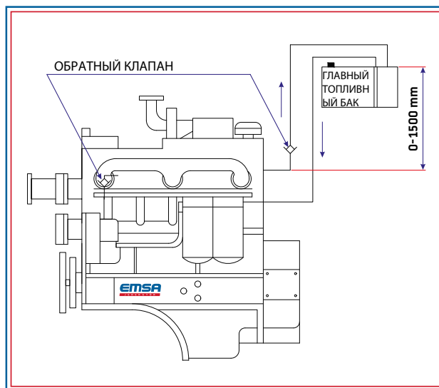
Рисунок-12b Топливный бак, установленный на высоте приблизительно более 1500 мм от линии обратной подачи топлива, и подсоединение обратного клапана
